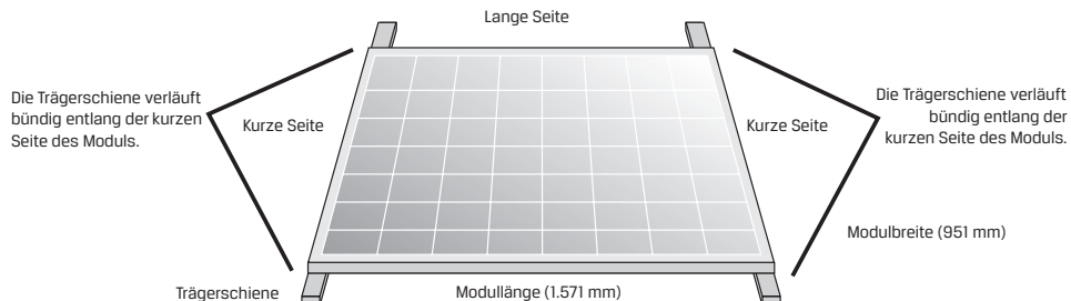
Abbildung 1: Endmontage
